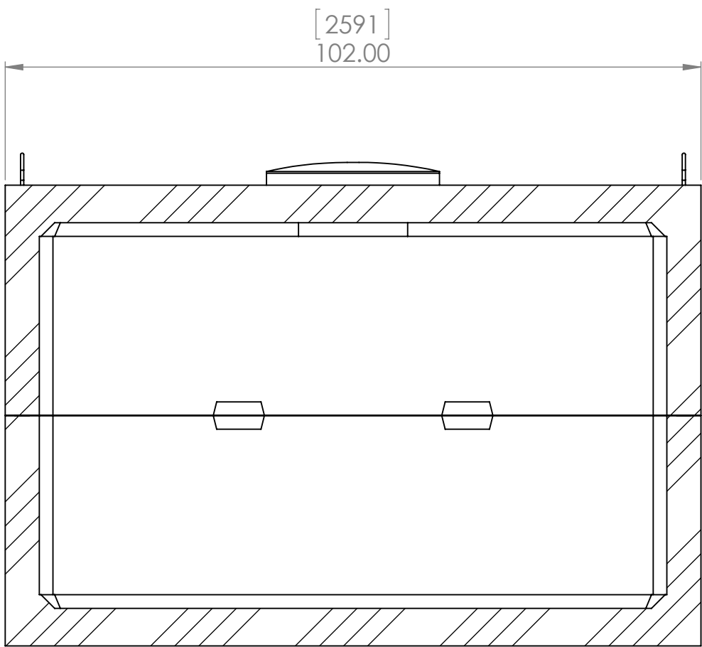
SECTION D-D
